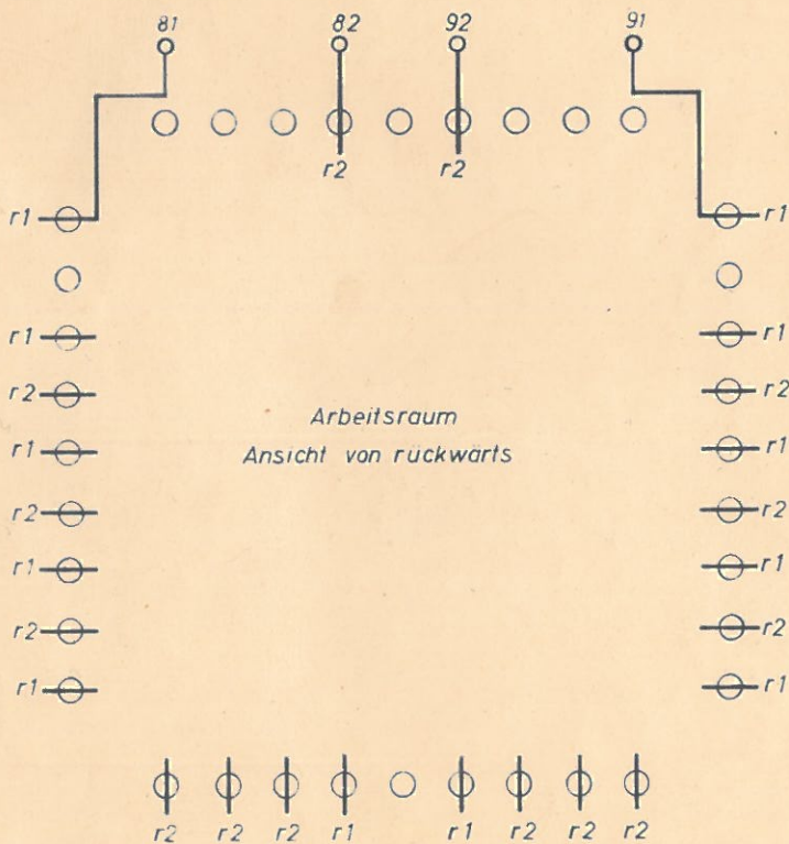
Schalter u Signalleuchten Ansicht von rückwärts
